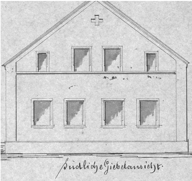
Zeichnung Giebelansicht aus Bauplan von 1880 // Quelle: Staatsarchiv Amberg
